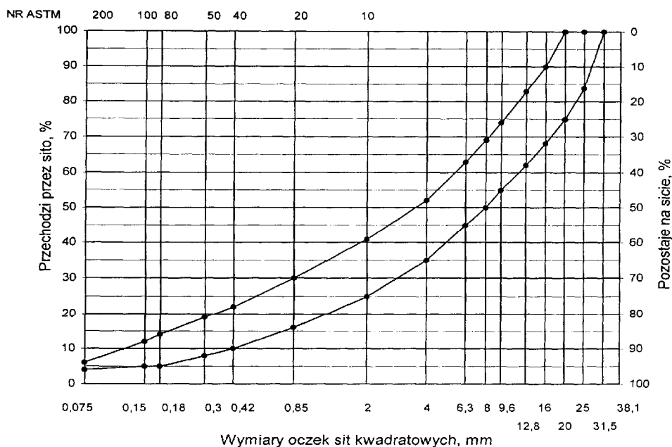
Rys. 4. Krzywe graniczne uziarnienia mieszanki mineralnej BA od 0 do 20 mm do warstwy wiążącej, wyrównawczej i wzmacniającej nawierzchni drogi o obciążeniu ruchem KR3
