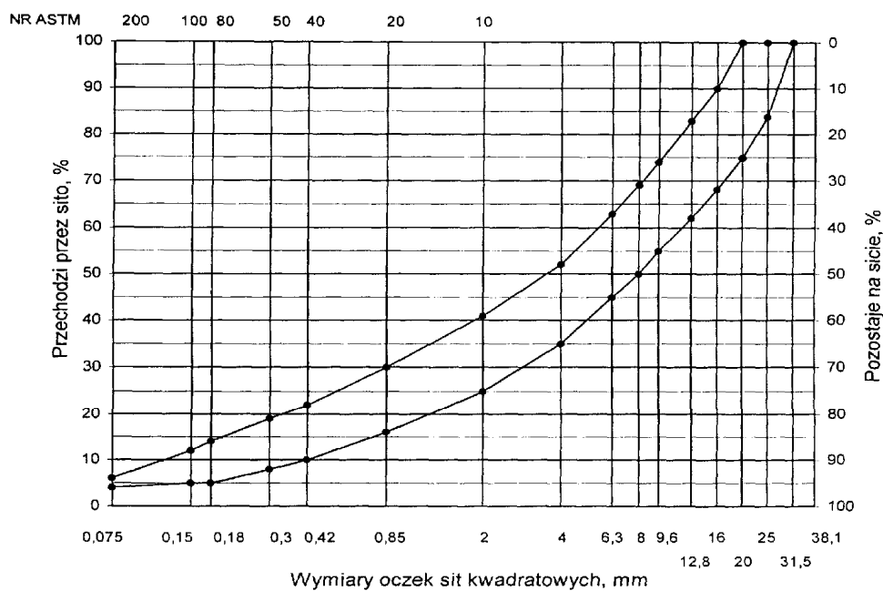
Rys. 3. Krzywe graniczne uziarnienia mieszanki mineralnej BA od 0 do 25 mm do warstwy wiążącej, wyrównawczej i wzmacniającej nawierzchni drogi o obciążeniu ruchem KR3
